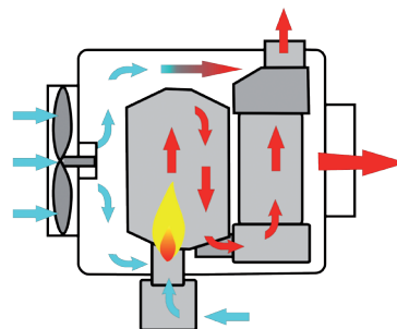
ISA 65 égő és kapcsoló doboz opcionális ventilátor sebesség szabályozóval.
